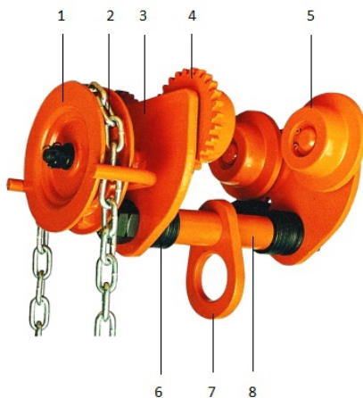
Рисунок 2. Устройство тележки
